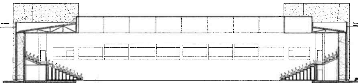
CORTE D-D
